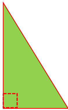
Retvinklet trekant
