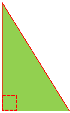
Retvinklet trekant
